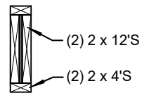
SECTION 'A - A'
